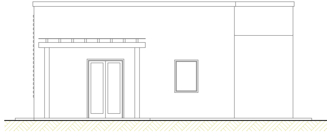
PROSPETTO SUD DI PROGETTO
