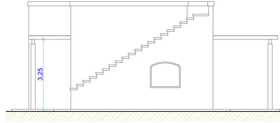
PROSPETTO OVEST DI PROGETTO
