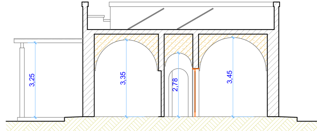
SEZIONE AA DI PROGETTO
