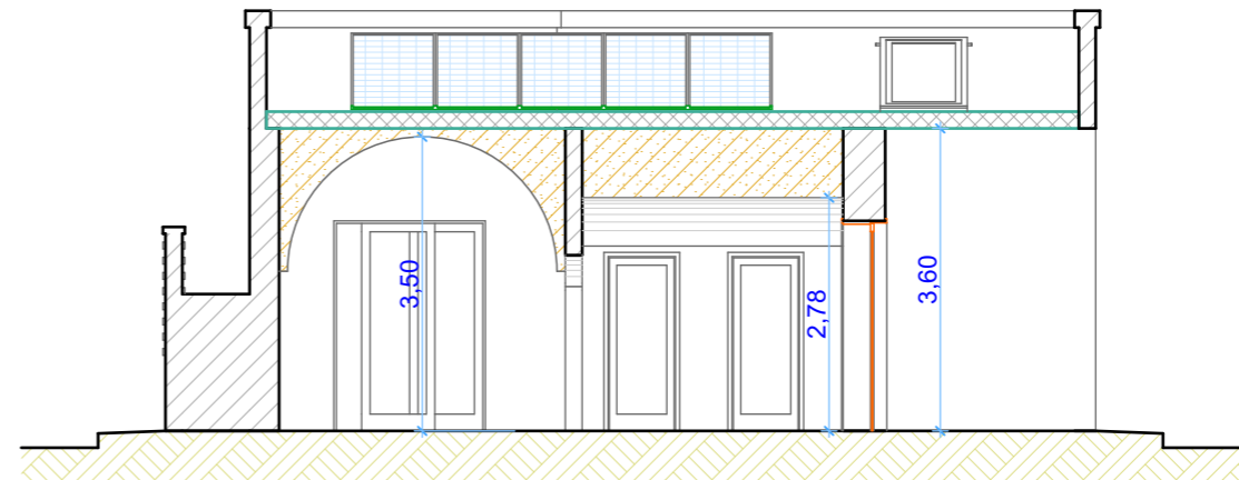
SEZIONE BB DI PROGETTO
