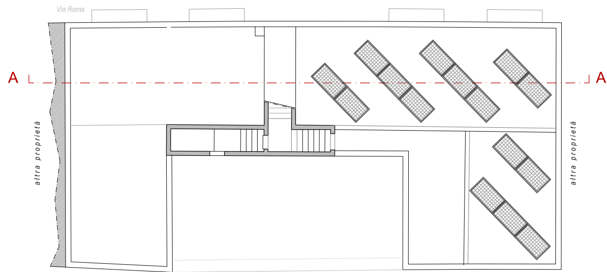
PIANO COPERTURA
