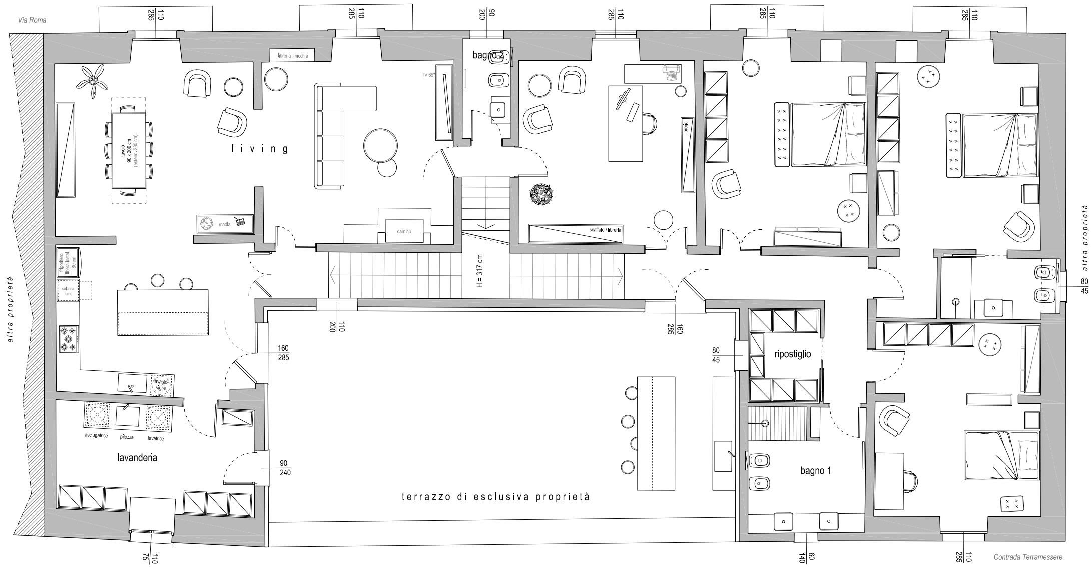
PIANO PRIMO scala 1:100
